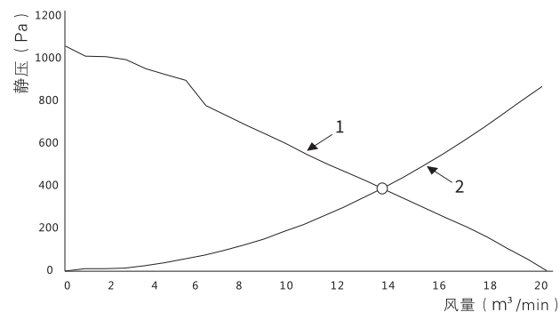
■ 空气性能特性曲线及阻力曲线
