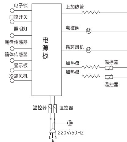
蒸烤箱部分电气原理图
