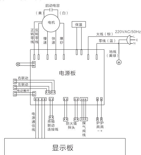
集成灶部分电气原理图
