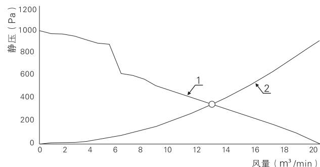
■ 空气性能特性曲线及阻力曲线
