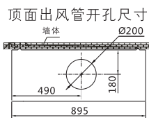
风管拉伸后尺寸
