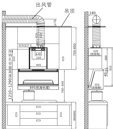
出风管走吊顶安装示意图
