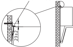
防跌挡块安装尺寸
