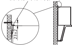
防跌挡块安装尺寸
