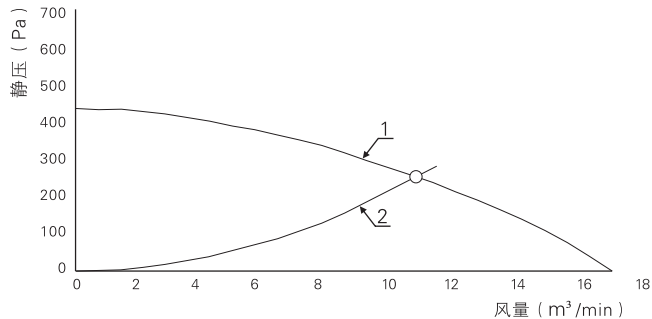
■ 空气性能特性曲线及阻力曲线
